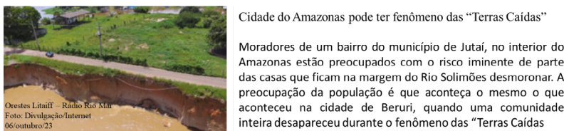
Figura 37 – Possível fenômeno das “terras caídas”
